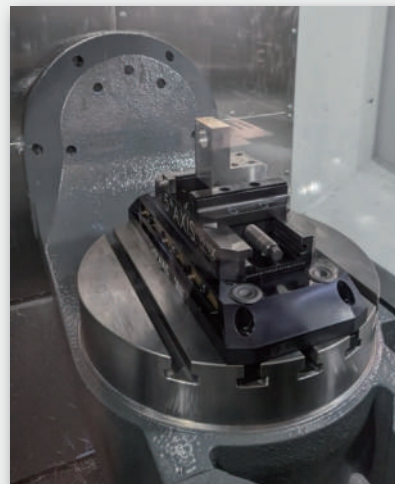
UMC-500と弊社取り扱いの 5th AXIS社製のバイス
