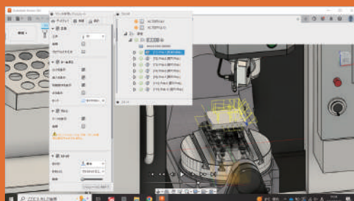
UMC-500用の加工パスを作成
